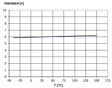
Figure 29: Vsenseh vs. Tcase
