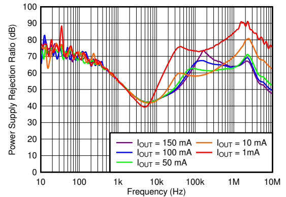
Figure 8-9. PSRR
