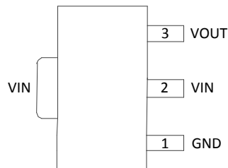
SOT89
